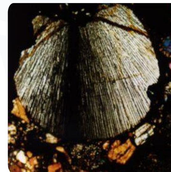
Пироксенска хондрула (хондрит)
